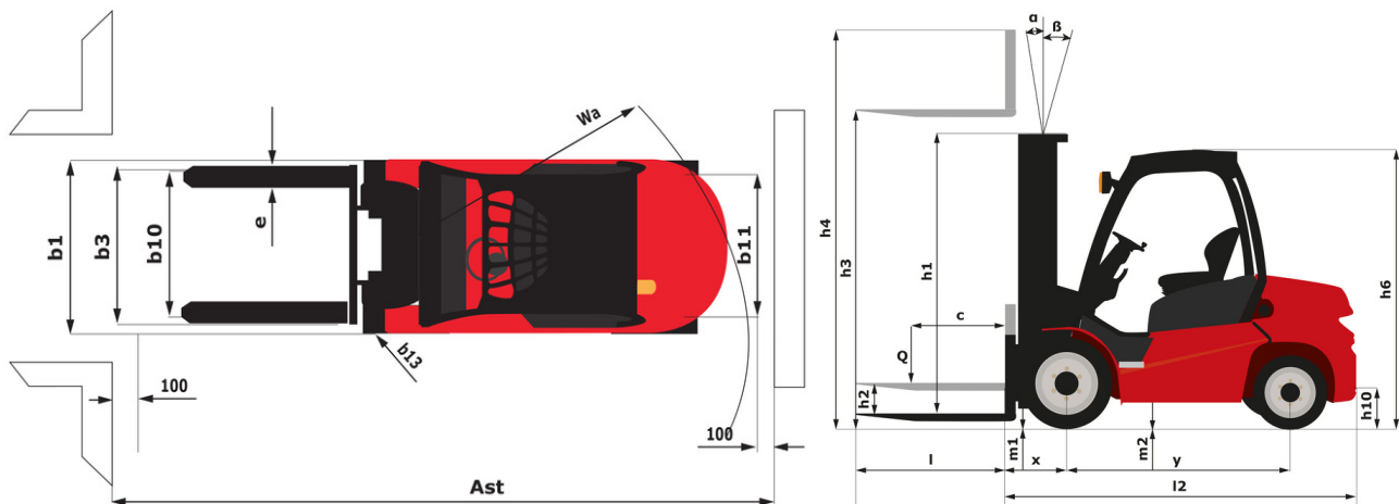
MI-X 80 D - 尺寸图
