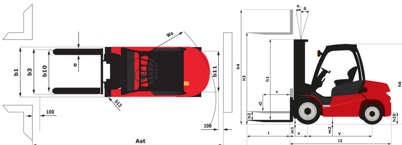
MI-X 60 D - 尺寸图
