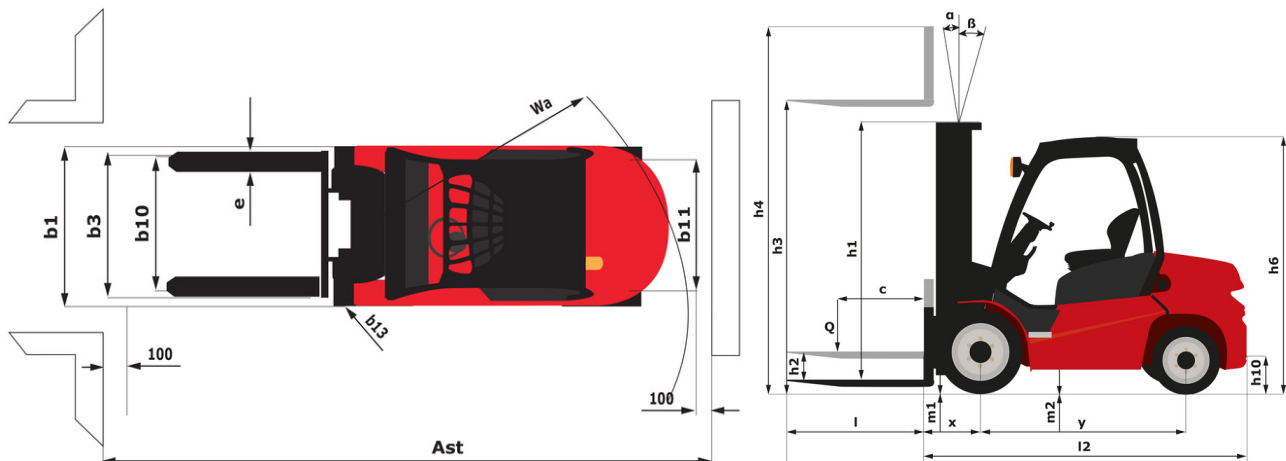
MI-X 35 D - 尺寸图
