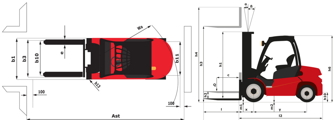
MI 50 LD ST5 FOB - 尺寸图
