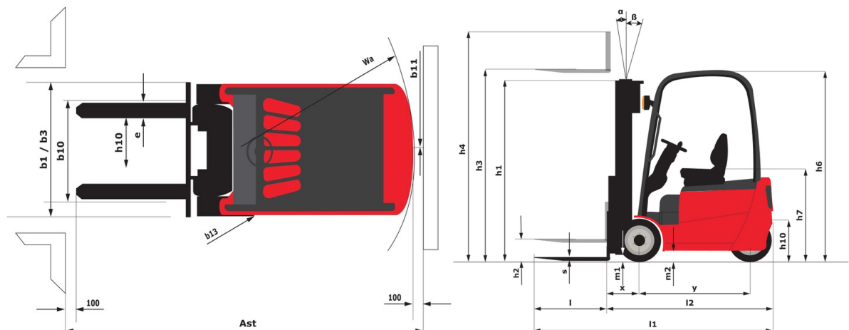
ME 445 FOB - 尺寸图
