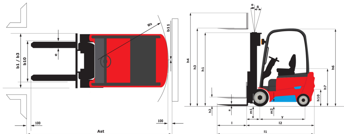
ME 430 LIFT - 尺寸图
