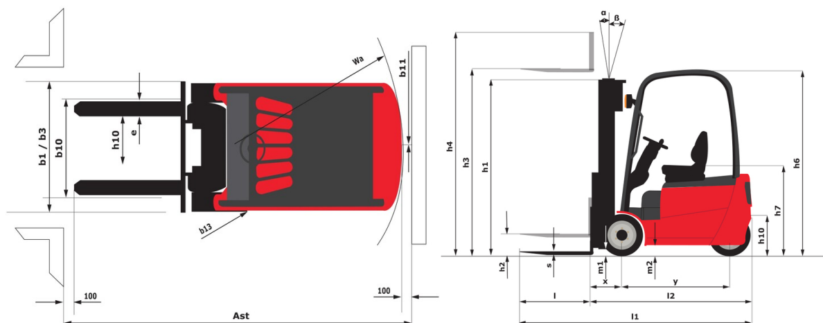
ME 425C FOB - 尺寸图
