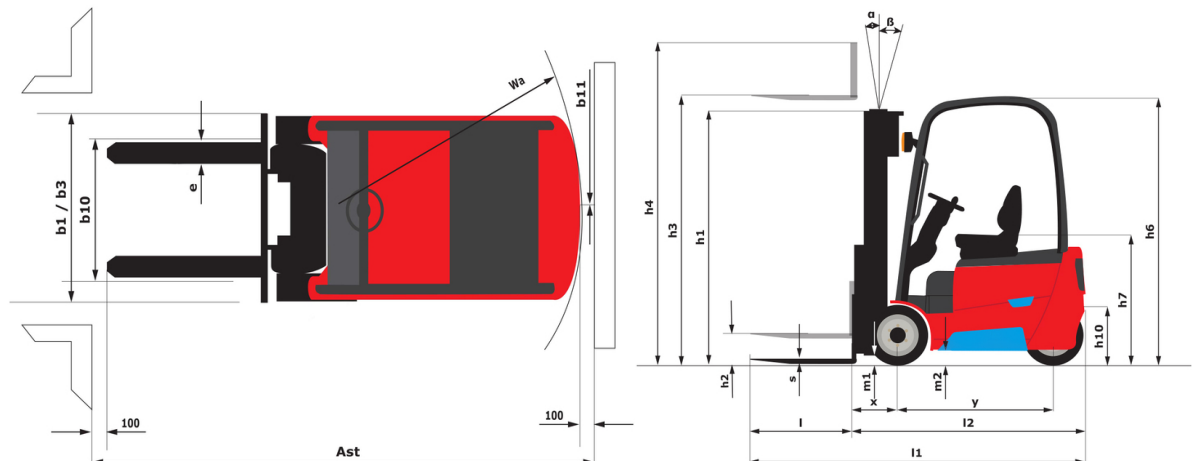
ME 316 LIFT - 尺寸图
