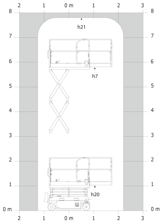
高空作业平台负载图表
