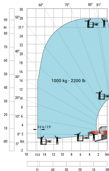
支腿完全打开 车身旋转 带 1000kg工作平台
