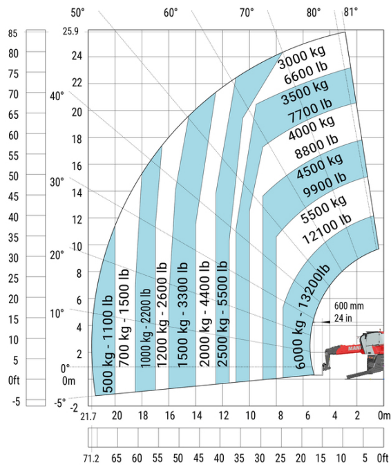
支腿打开 带货叉 CAF 公制
