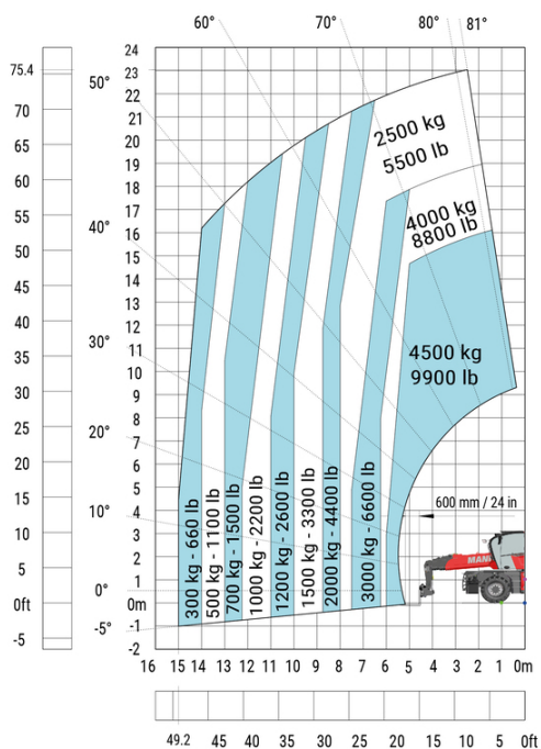
机器在轮胎上 带货叉
