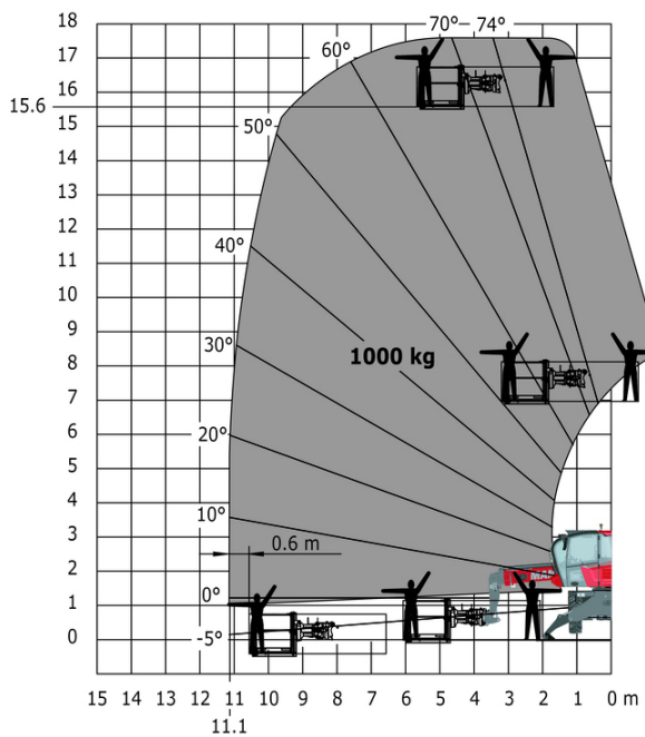
支腿完全打开 车身旋转 带 1000 kg工作平台
