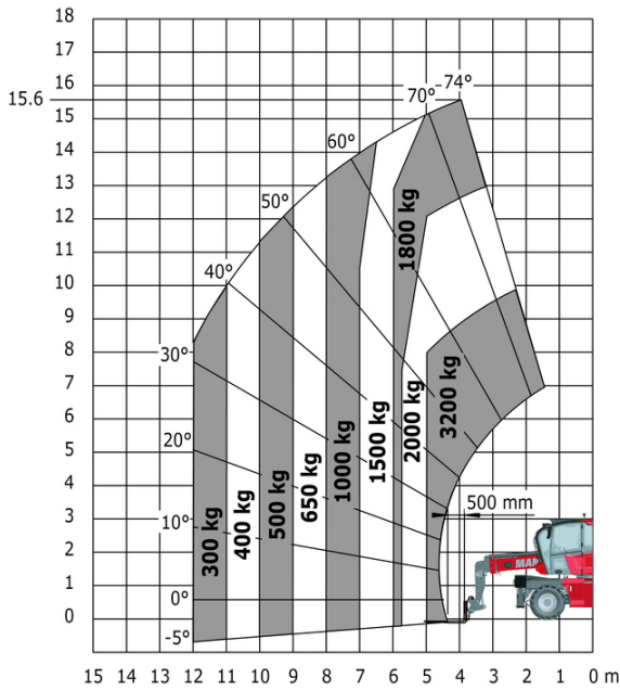
机器在轮胎上 带货叉
