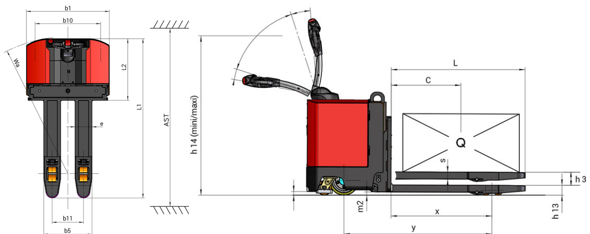
EP 730 - 尺寸图
