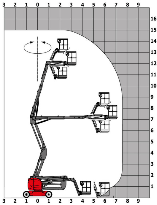
载荷曲线表
