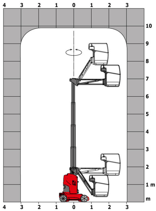
高空作业平台负载图表
